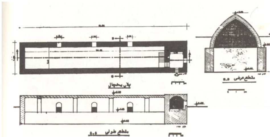
تصویر شماره ۱۰: نقشه یخچال دو قوز پله، ارومیه
