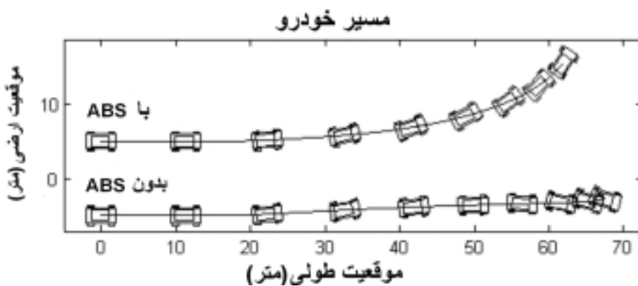
شکل ۱۱ ترمز در حال دور زدن
