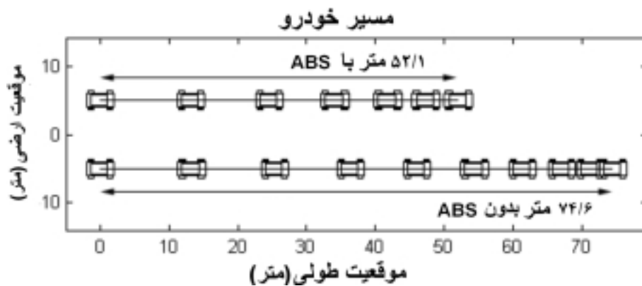
شکل ۱۰ ترمز در مسیر مستقیم
