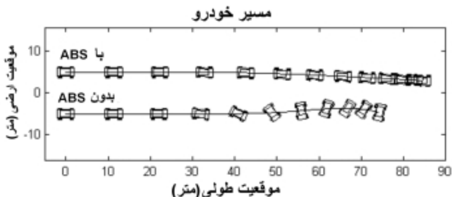
شکل ۱۲ ترمز در جاده‌ای با ضریب اصطکاک دوگانه
