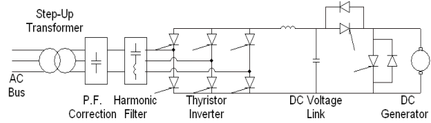
شکل 10: آرایش ژنراتور DC با دو چاپر افزایشنده (DC/AC)
