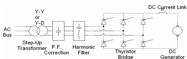
شکل 1: ژنراتور DC همراه با سیستم اینورتری (DC/ AC)
