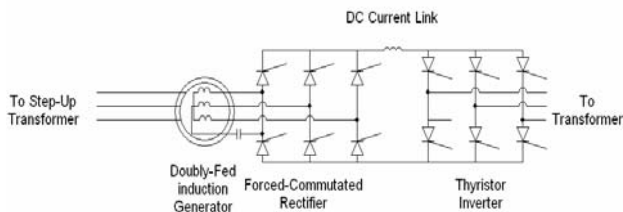
شکل 6: آرایش ژنراتور القایی دوسو تغذیه و یکسوساز کموتاسیون اجباری
