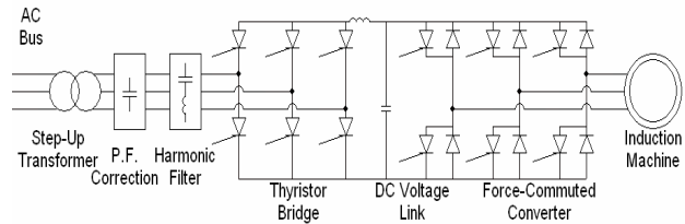
شکل 11: آرایش ژنراتور القائی با رابط ولتاژ DC و مبدل (AC/DC/AC)
