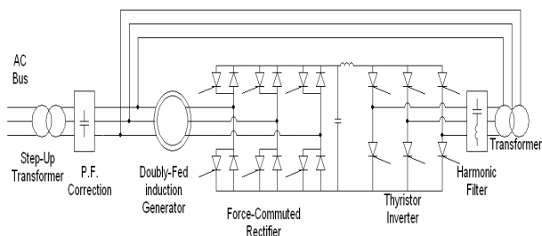
شکل 7: آرایش ژنراتور القایی دوسو تغذیه با رابط ولتاژ DC
