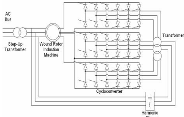
شکل 9: کاربرد ژنراتور آسنکرون دوسو تغذیه و سیکلوکانورتر
