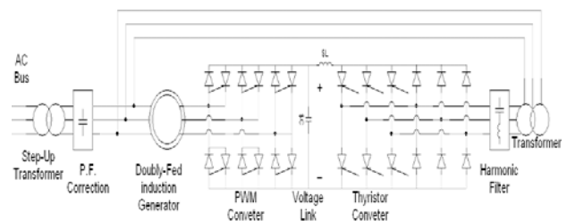
شکل 8: ژنراتور القایی دوتغذیه بادو حالت کار سرعت فوق و تحت سنکرون
