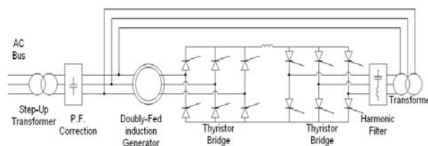
شکل 5: ژنراتور القایی دوسو تغذیه با اینورتر / یکسوساز (AC/DC/AC)
