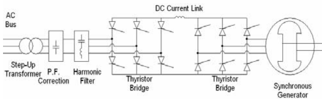
شکل 4: آرایش ژنراتور سنکرون با سیستم اینورتر (DC/AC)
