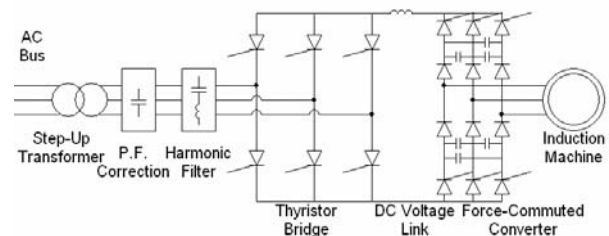
شکل 12: آرایش ژنراتور القائی با رابط جریان DC و مبدل AC/DC/AC
