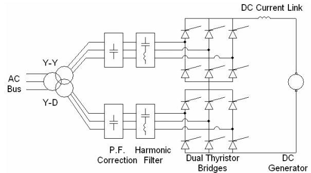
شکل 2: آرایش ژنراتور DC همراه با سیستم اینورتری دوگانه
